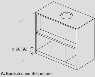
A: Bereich ohne Scharniere
