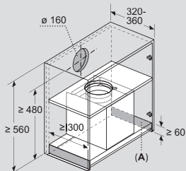
A: Bereich ohne Scharniere
