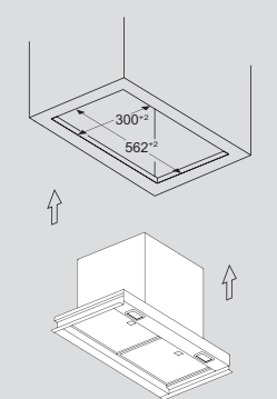
Einbaubeispiel in Möbelausschnitt
