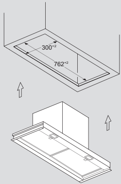
Einbaubeispiel in Möbelausschnitt
