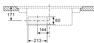
Vorderansicht – Geräteausschnitt für ungefasste Umluft
