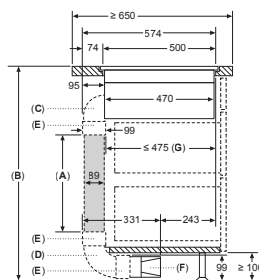
Vorderansicht – Geräteausschnitt für ungefasste Umluft
