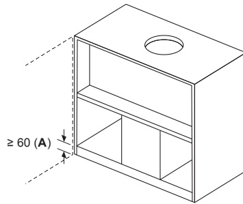
Einbaubeispiel mit Gewürzregal
