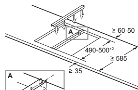
Montagesatz (HEZ394301) für Domino
